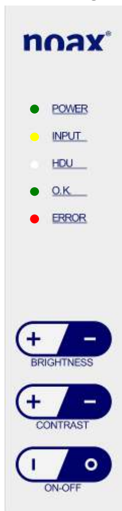
Abb. 2 Anzeige- und Bedienelemente S12
